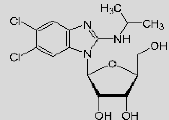
Benzimidazole riboside
